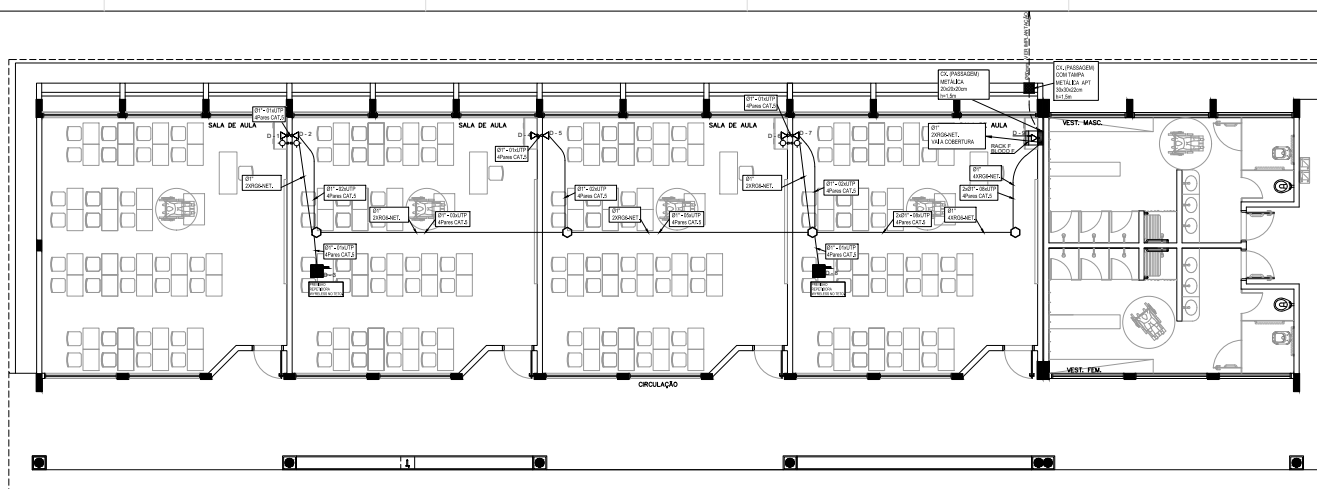
1 PLANTA BAIXA - BLOCO F SEM ESCALA
