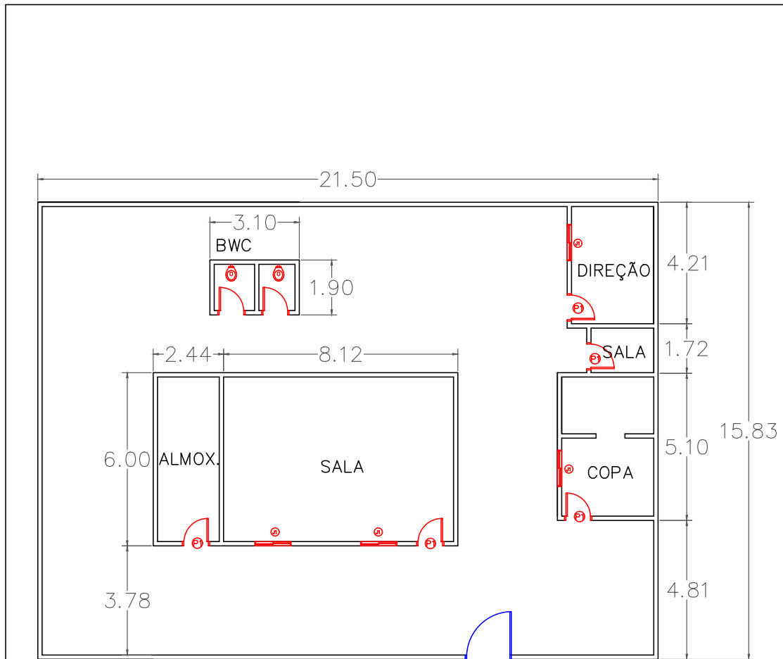
PLANTA BAIXA ESCOLA JOEL CAETANO DOS REIS
