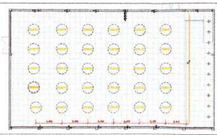
ILUMINAÇÃO AUDITORIO F1 1:150
