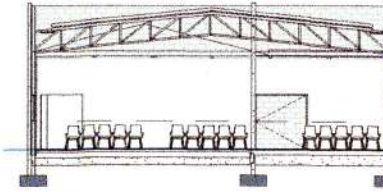
CORTE 01 F1 1:100
