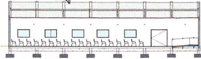
CORTE 02 F1 1:100
