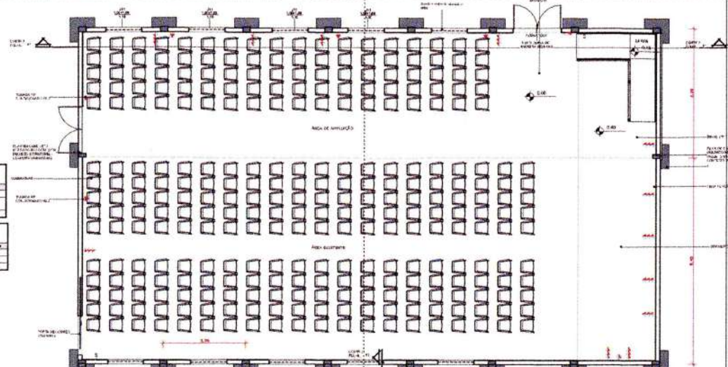
PLANTA BAIXA AUDITORIO F1 1:75
